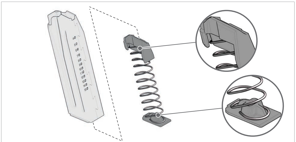
Abb. 73: Montageposition der Einzelteile
