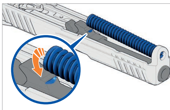
Abb. 68: Schließfeder abstützen
