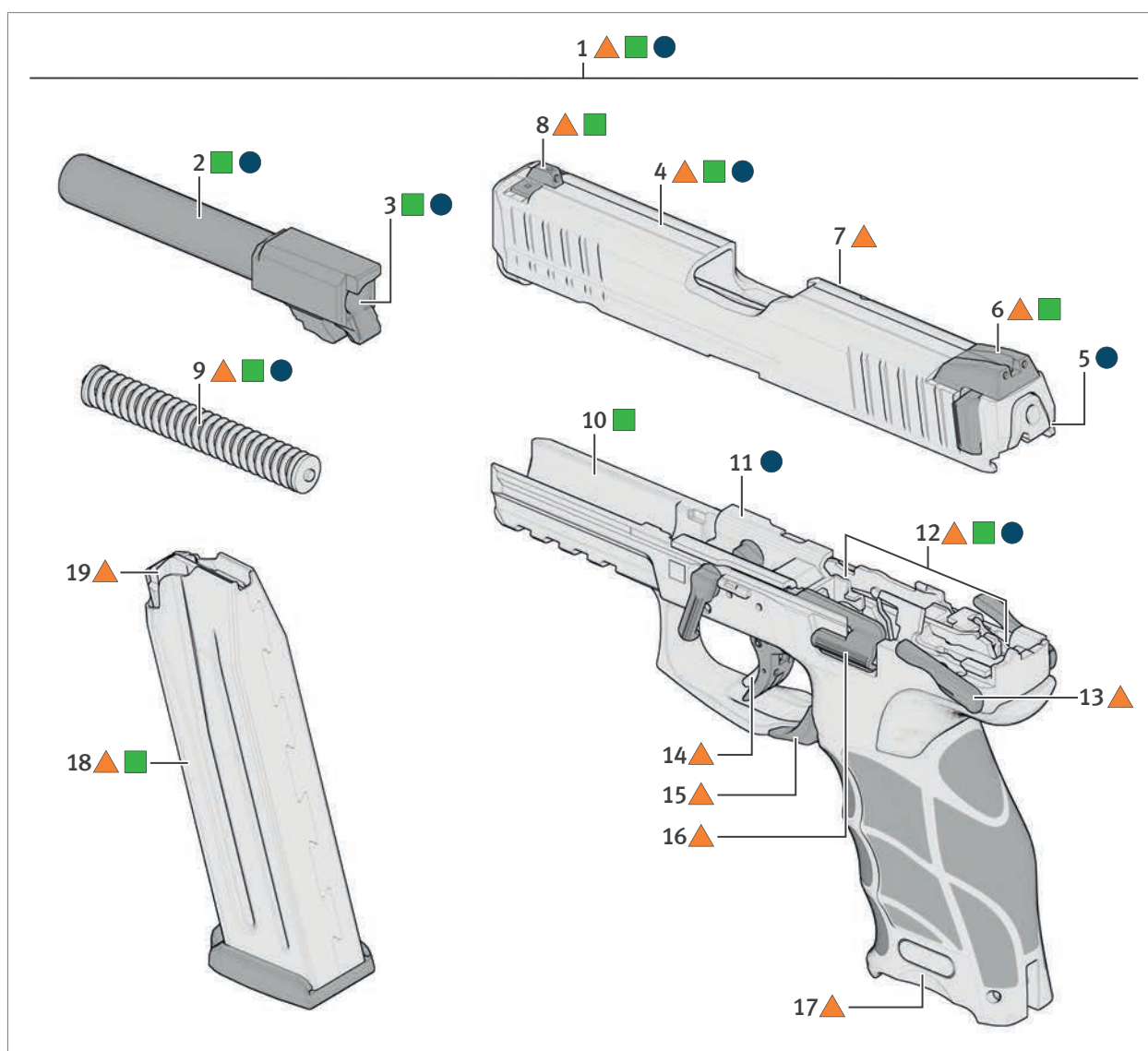
Abb. 58: Übersicht der Wartungsstellen
