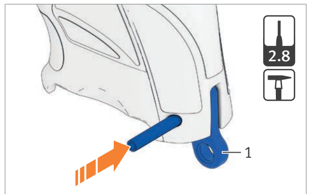
Abb. 29: Aufnahme für Sicherungsschnur einsetzen
