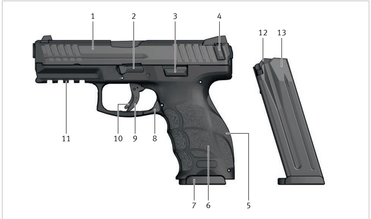
Abb. 4: Ansicht von links
