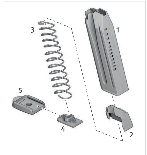
Abb. 72: Magazin montieren
