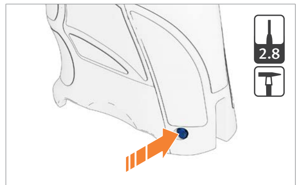
Abb. 26: Spannstift für Griff Rücken austreiben
