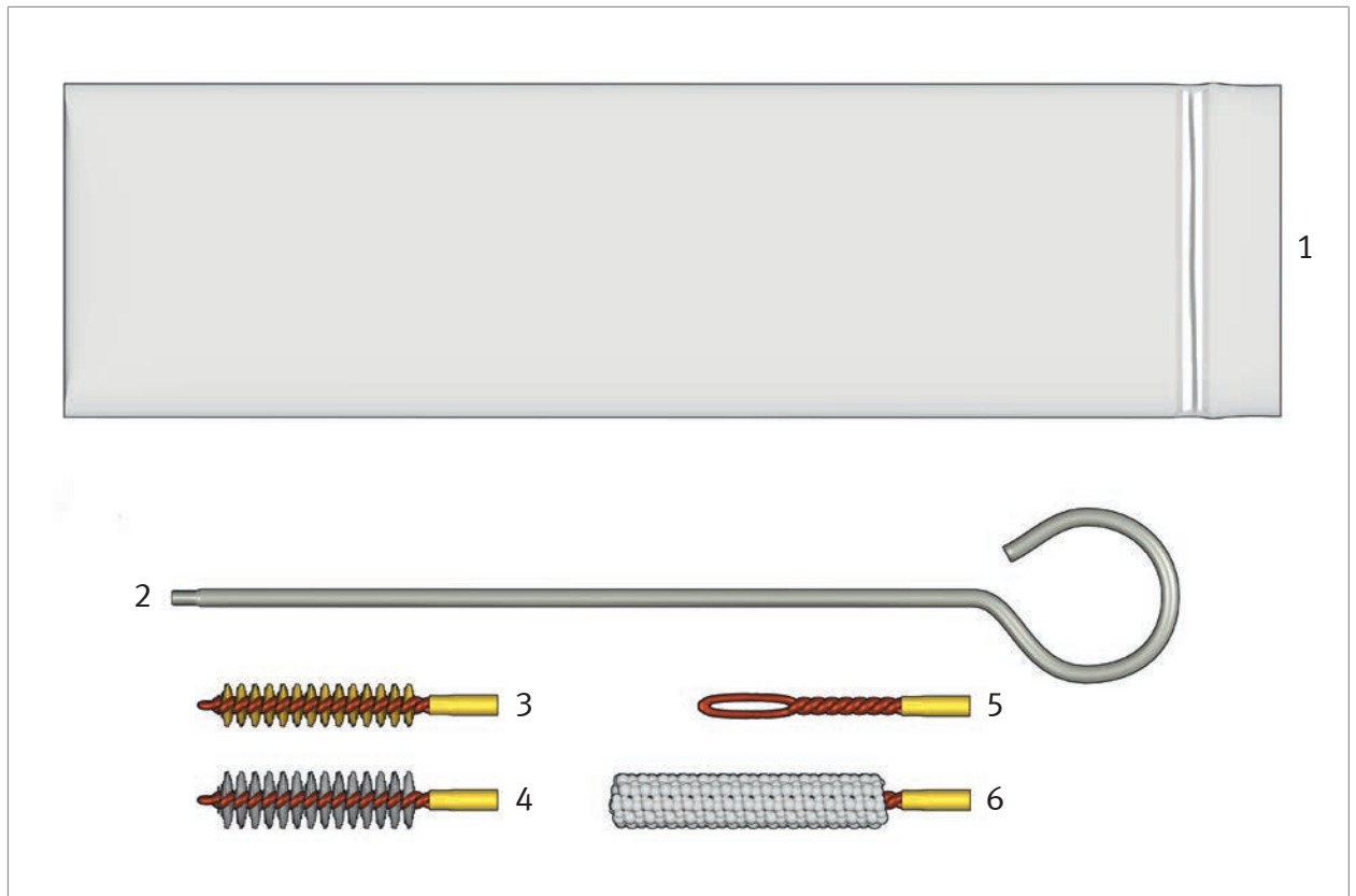
Abb. 18: Reinigungsgerät (Ident.-Nr. 987837)
