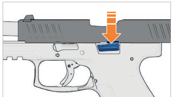
Abb. 24: Verschlussfanghebel nach unten drücken
