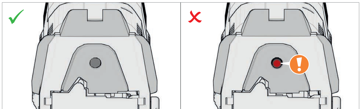
Abb. 20: Spannanzeige für Schlagbolzen
