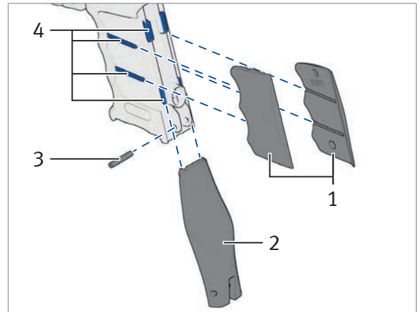
Abb. 25: Griff Rücken und Griffschalen
