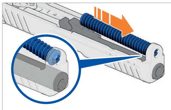
Abb. 67: Schließfeder einsetzen
