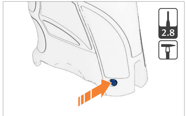
Abb. 28: Spannstift für Griff Rücken austreiben
