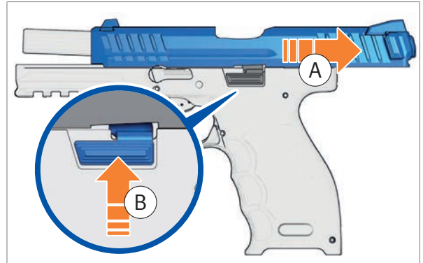
Abb. 23: Verschluss arretieren
